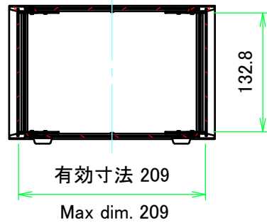
A-A ( 1 : 6 )
