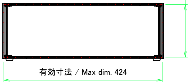
C-C ( 1 : 6 )
